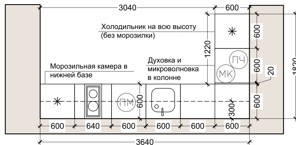
План расположения мебели
