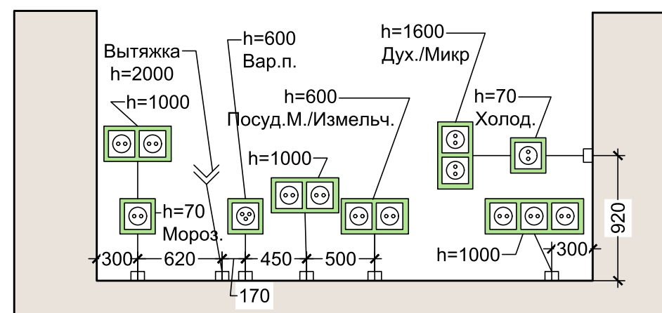
План электрики
